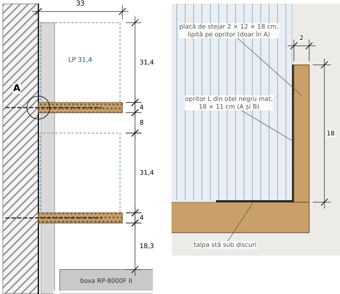
SECȚIUNE (1:15)
