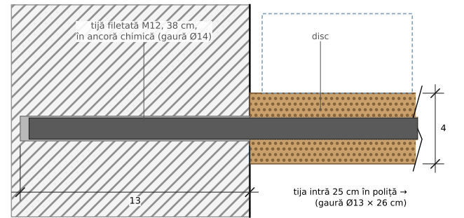
DETALIU A - prinderea ascunsă (1:3)
